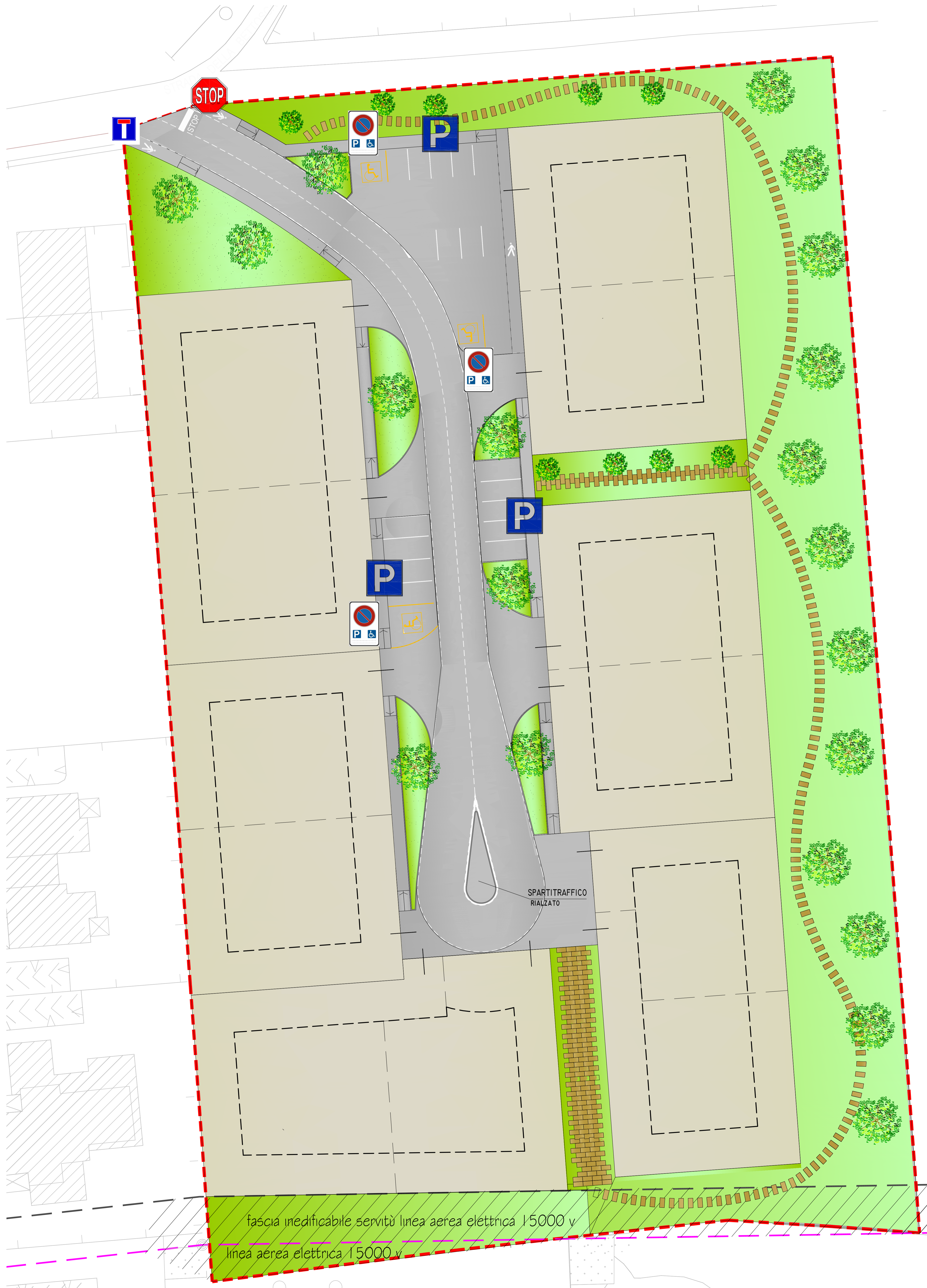
PLANIMETRIA GENERALE - SEGNALETICA SCALA 1:200
