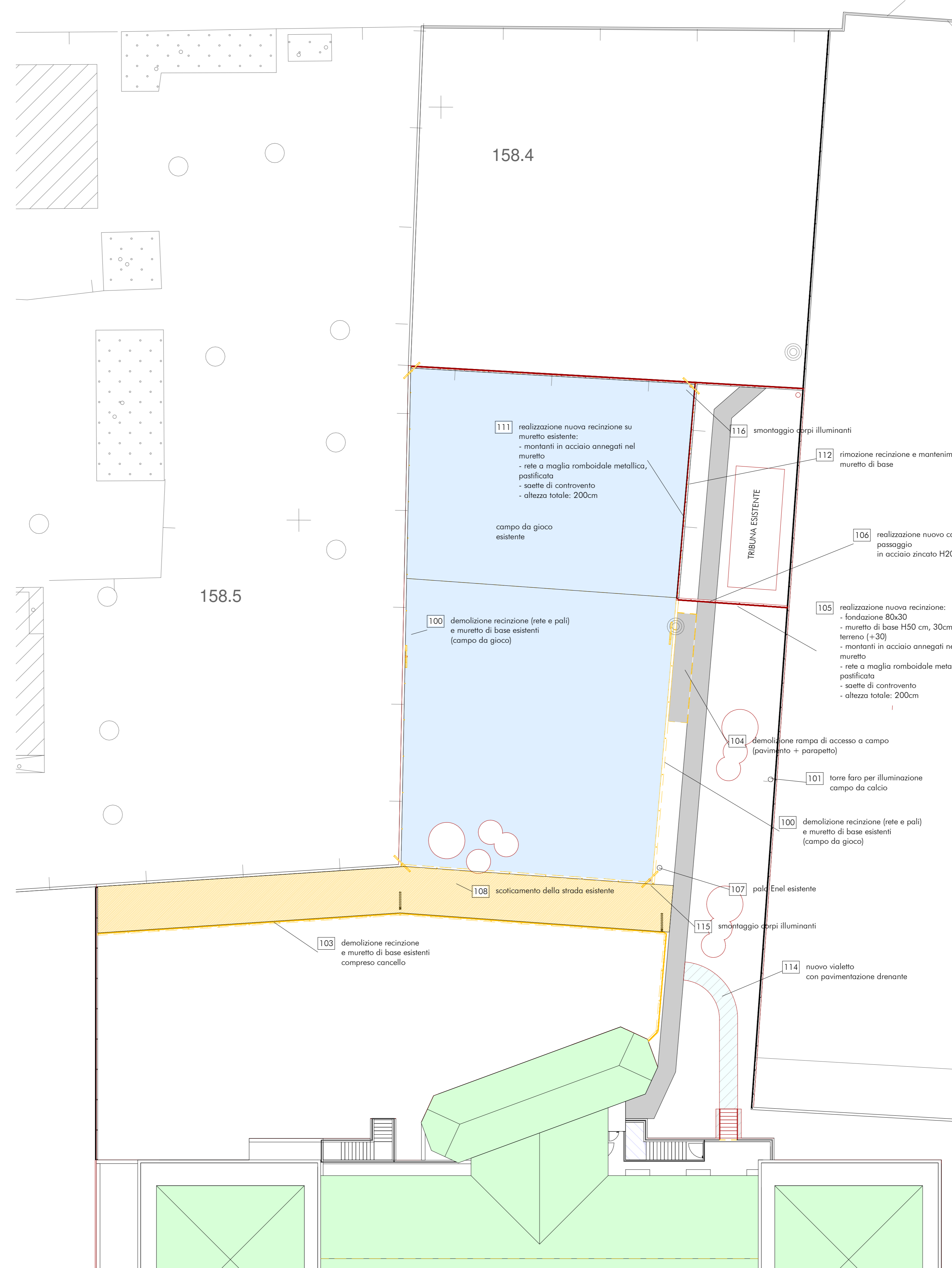
OPERE ESTERNE - DEMOLIZIONI COSTRUZIONI Scala 1:200
