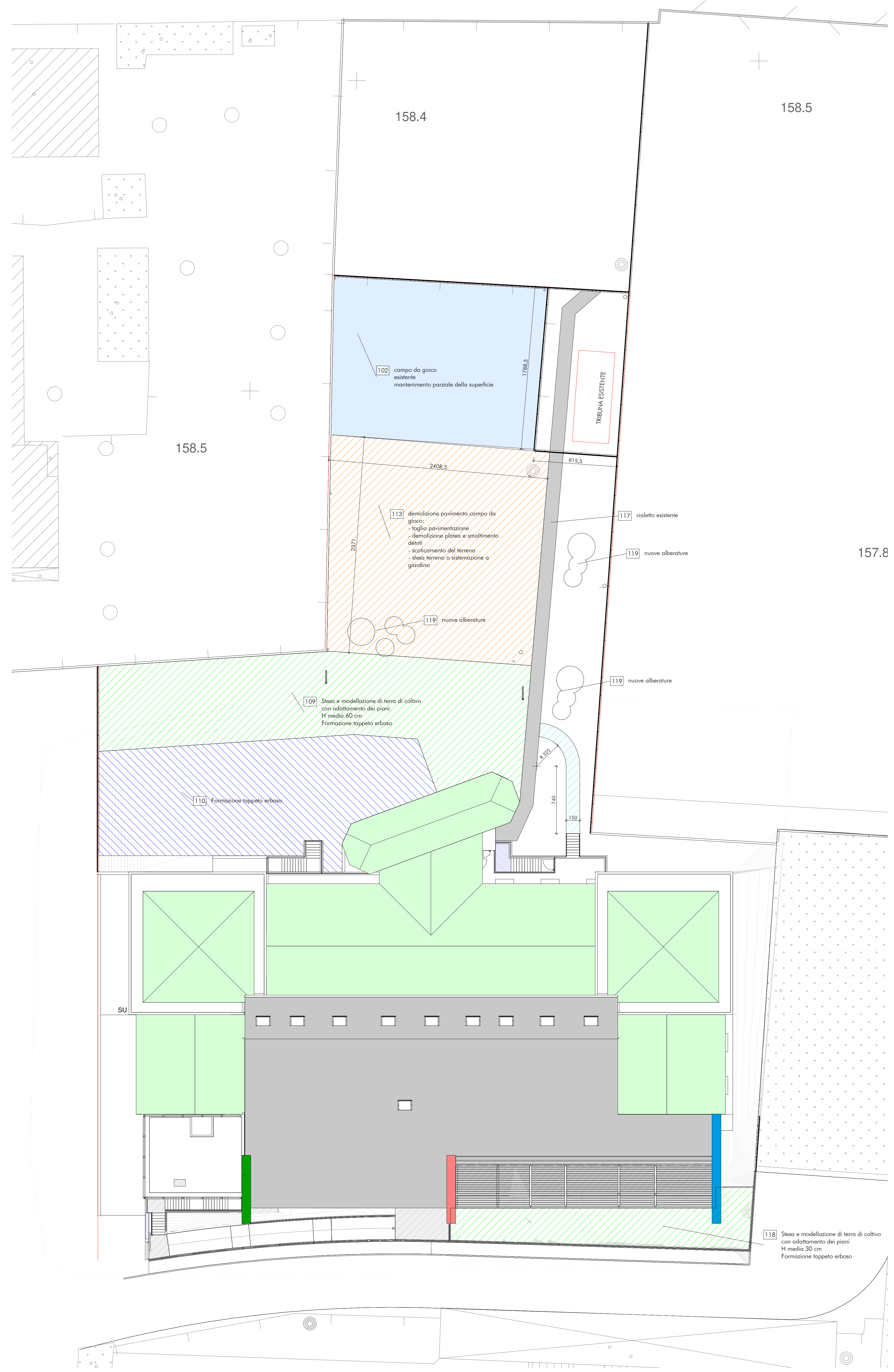
OPERE ESTERNE - STATO DI PROGETTO
